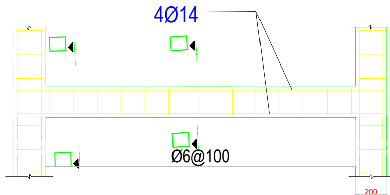
បង់ស ស ដែក ធីម គ្រឹះ GB2, GROUND BEAM GB2 មាត្រដ្ឋាន ១:២០
