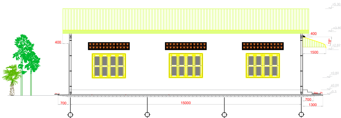
មើលពីឆ្វេង Left View មាត្រដ្ឋាន ១០០ Scale 1/100
