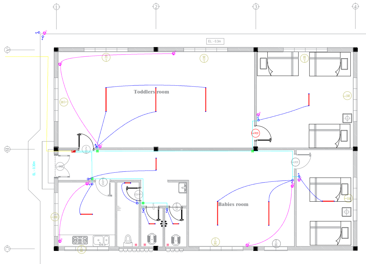
លំអិតប្រព័ន្ធគ្រឡូកក្នុងអាគារ រោងចក្រ ១០០
