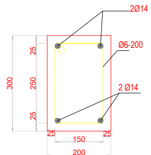
១១១ មាត្រដ្ឋាន ១:១០
