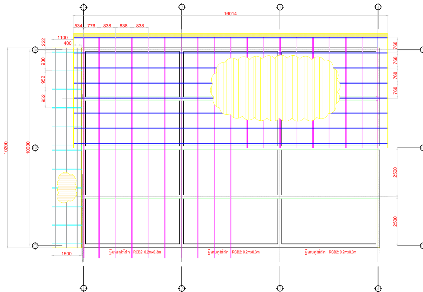
បង់ស មូលដ្ឋានដីបូល Roof Structure មាត្រដ្ឋាន ១:១០០ Scale 1/100
