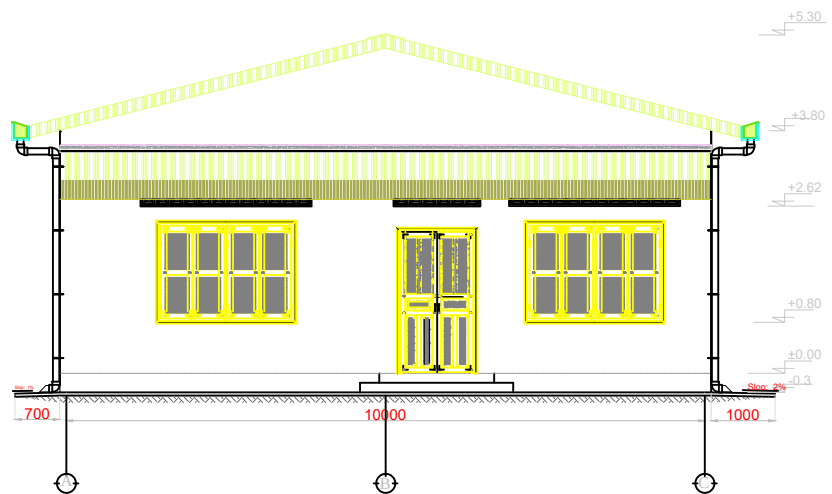
មើលពីមុខ Front View មាត្រដ្ឋាន ១:១០០ Scale 1/100
