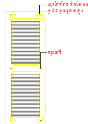
មើលពីខាងក្នុង មាត្រដ្ឋាន ១:២៥
