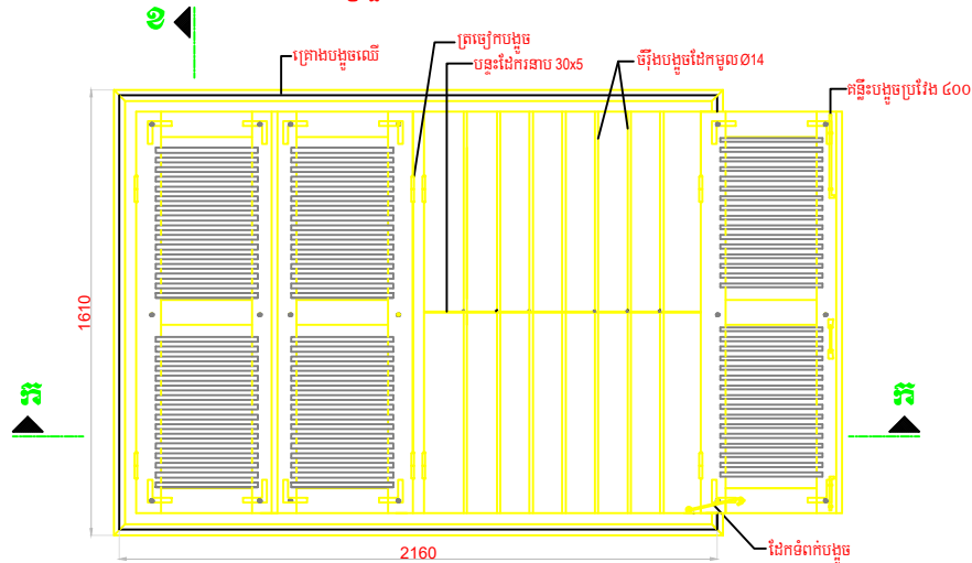
មើលពីខាងក្នុង មាត្រដ្ឋាន ១:២៥
