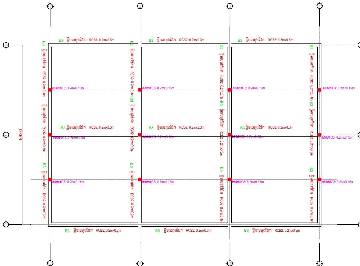
បង់សស C3 និង ឆ្នើម B3 នៅកម្រិត 3.8m មាត្រដ្ឋាន ១:១០០ Scale 1/100
