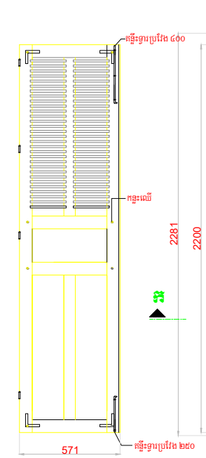
មើលពីខាងក្នុង មាត្រដ្ឋាន ១:២៥
