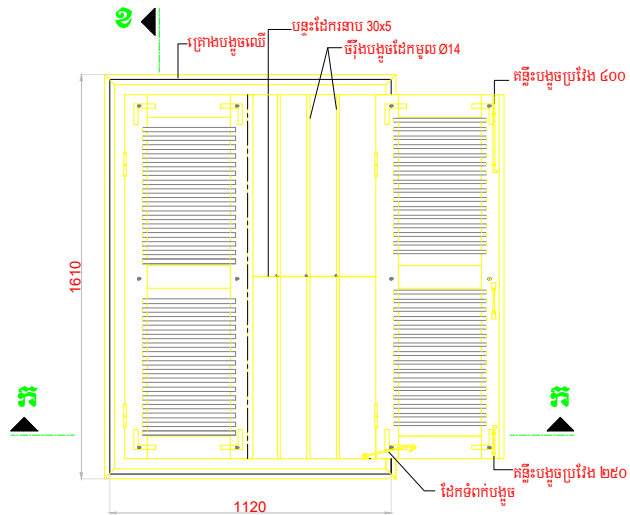
មើលពីខាងក្រៅបង្អួច W2 មាត្រដ្ឋាន ១:២៥
