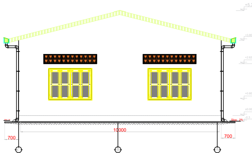
មើលពីក្រោយ Rear View មាត្រដ្ឋាន ១:១០០ Scale 1/100
