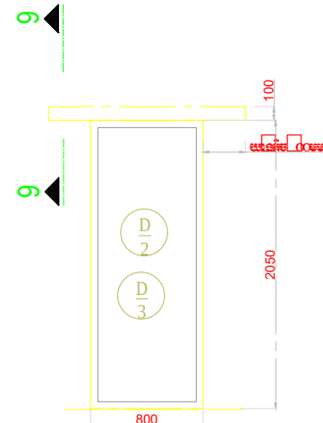
ផ្ទាំងបង្ហាញលើទ្វារជញ្ជាំងកំរាស់ ១០០មម មាត្រដ្ឋាន ១:២០
