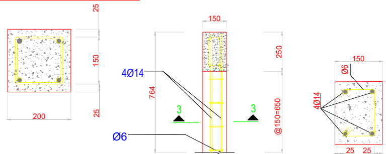
សរសៃក្បាល KING POST C3 SCALE 1:20
