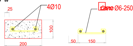
ផ្ទាំងបង្ហាញលើទ្វារជញ្ជាំងកំរាស់ ២០០មម មាត្រដ្ឋាន ១:២០
