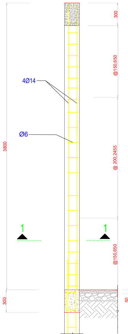
សរសៃ C1 និង ក្បាលសរសៃ C1 COLUMN C1 SCALE 1:25
