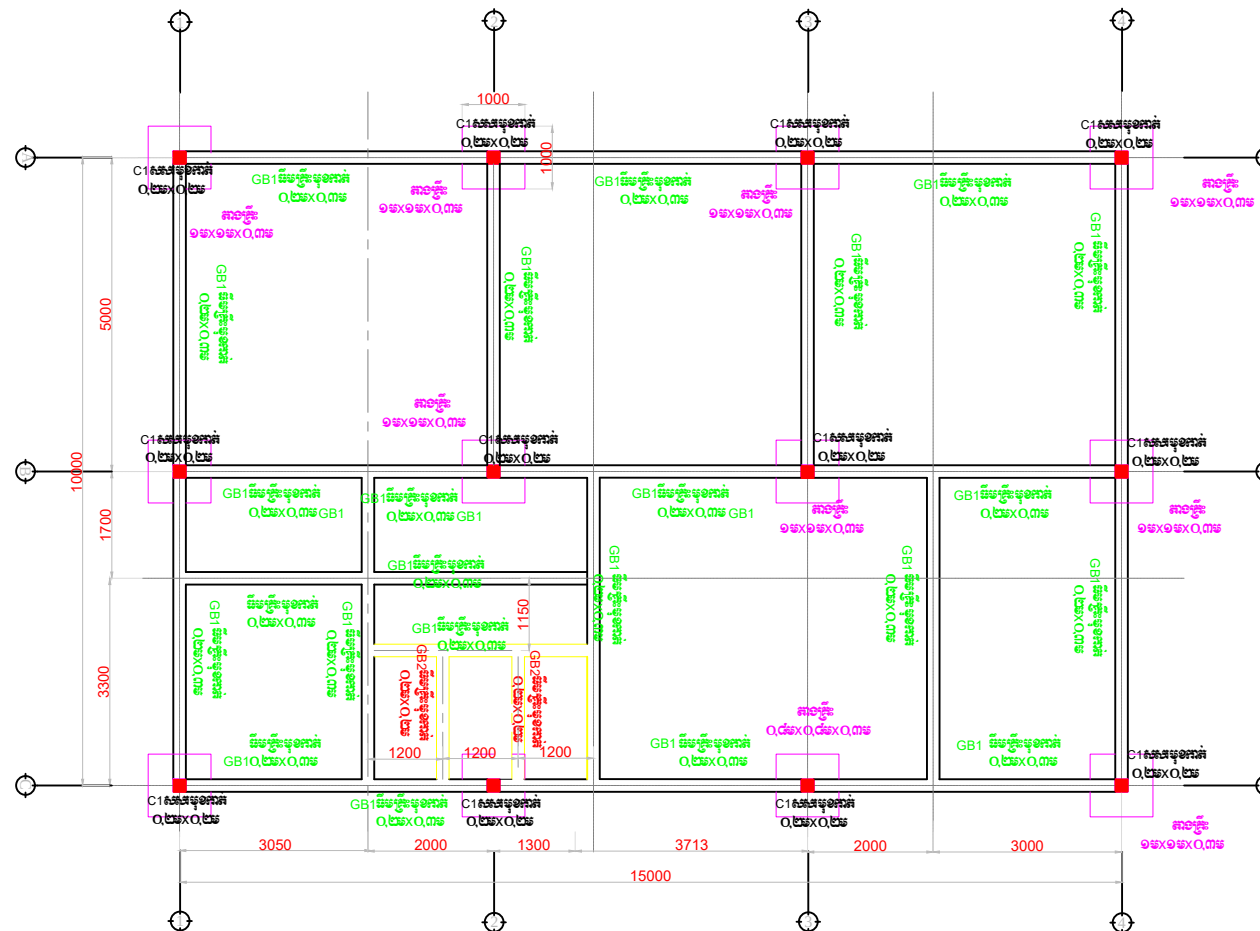
ប្លង់សរសេរ C1 ឆ្អឹង ឆ្អឹង GB1;GB2 ដើមគោល Groun Beam; Column; Footing កម្រិតទី ១ ១០០ Scale 1/100
