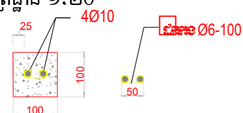
ព្រះ៩-៩ ផ្ទាំងបង្ហាញលើទ្វារទាំងអស់ ជញ្ជាំងកំរាស់ ១០០មម
